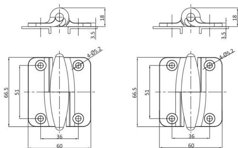
R型 (右裝) Version R(Right) B-2115-76604-R
