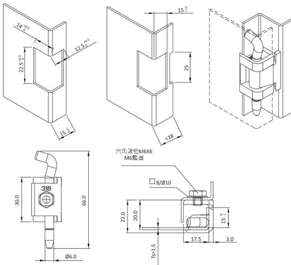
180°不鏽鋼SUS 316鉸鏈,不鏽鋼銷釘 180° hinge SUS 316, pin SUS 304
