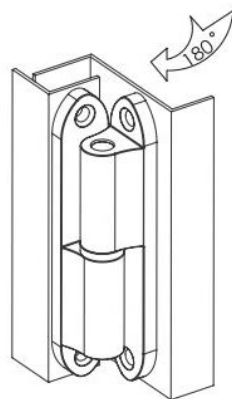
安裝示意
