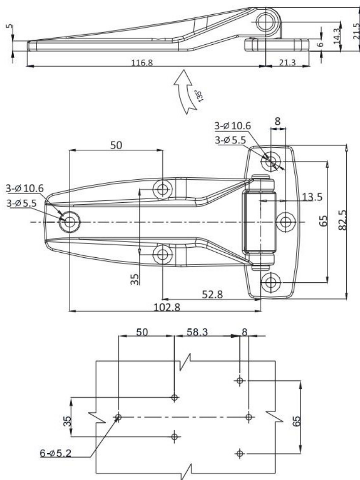
開孔尺寸 Panel Cutout
