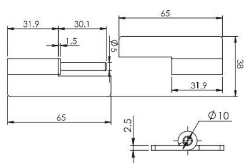
BS-3865-2L 右裝
