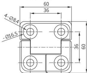
M8沉頭螺絲固定 Countersunk Screw M8
