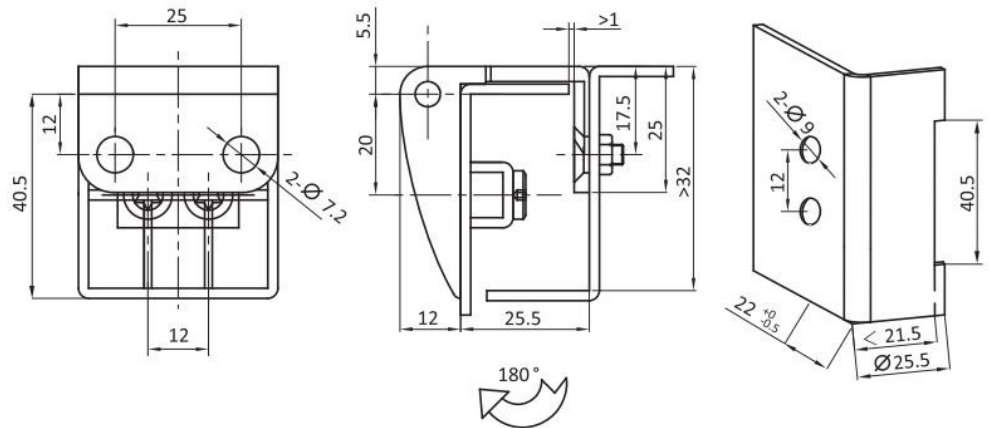
開孔尺寸 Panel cutout
