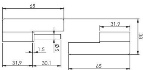
BS-3865-1R 左裝
