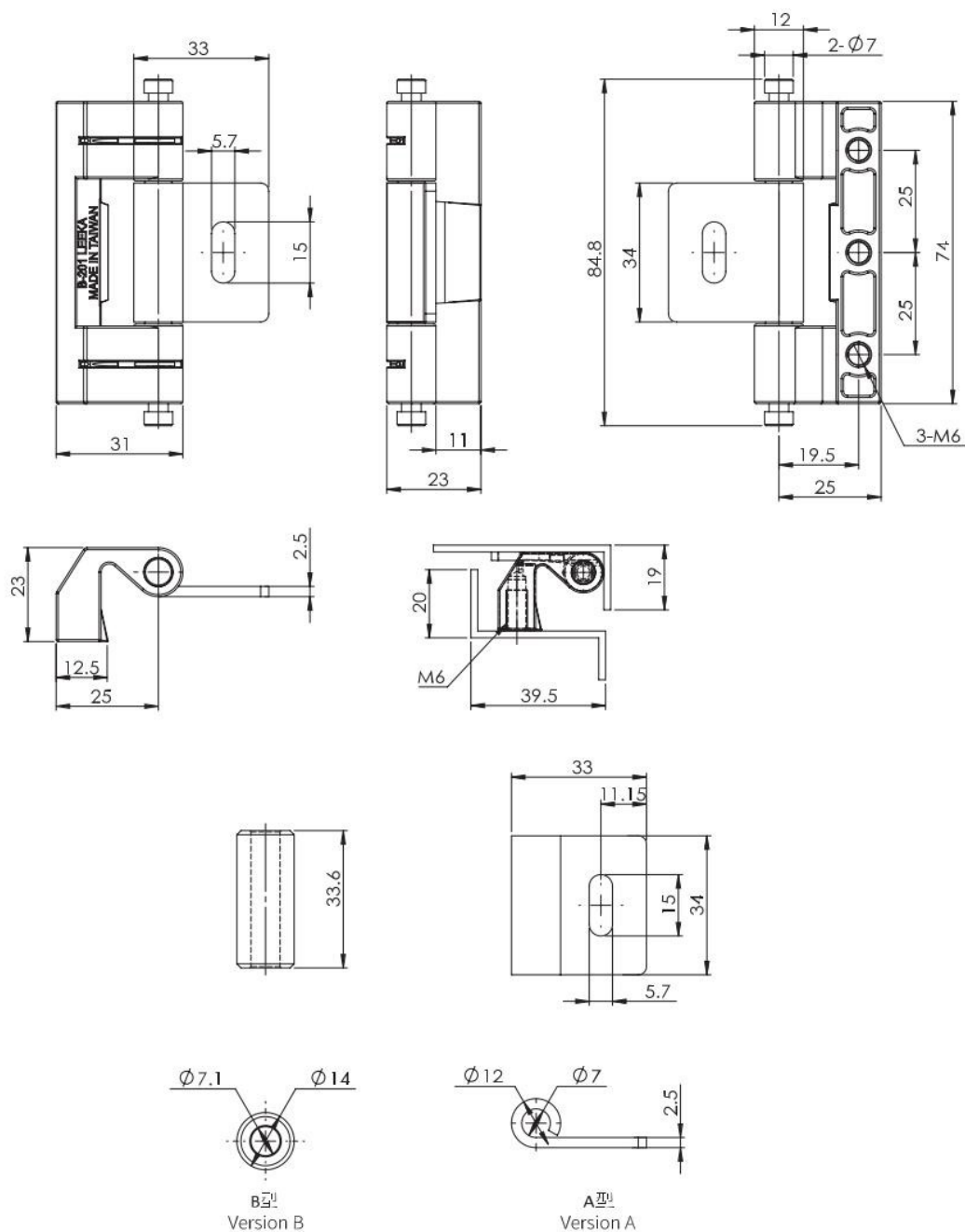
後鈕固定片
