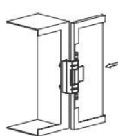
安裝示意二
