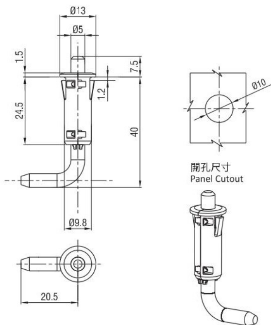
黑色PA鉸鏈，鋅合金銷軸 Black PA hinge, zinc die pin shaft
