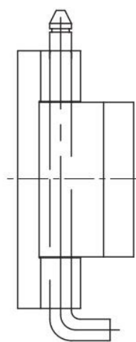
焊接固定型 Weld on version
