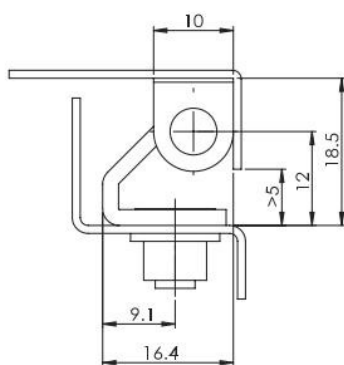
安裝示意2
