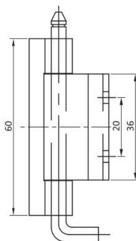
螺絲固定型 Screw on version
