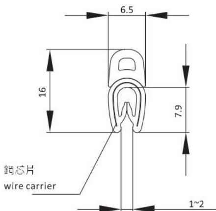
黑色發泡EPDM密封膠條 Sponge-rubber,Black EPDM gasket
